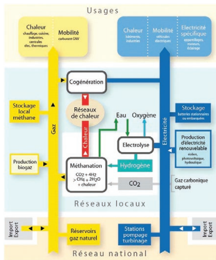
Figure 6 : processus de méthanation intégré dans le système énergétique national. Source : Négawatt
