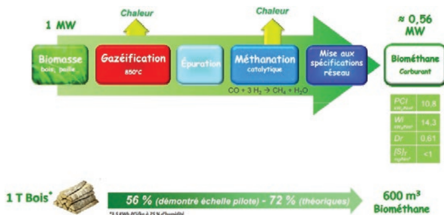
Figure 4 : Bilan énergétique du biométhane issu du bois.
