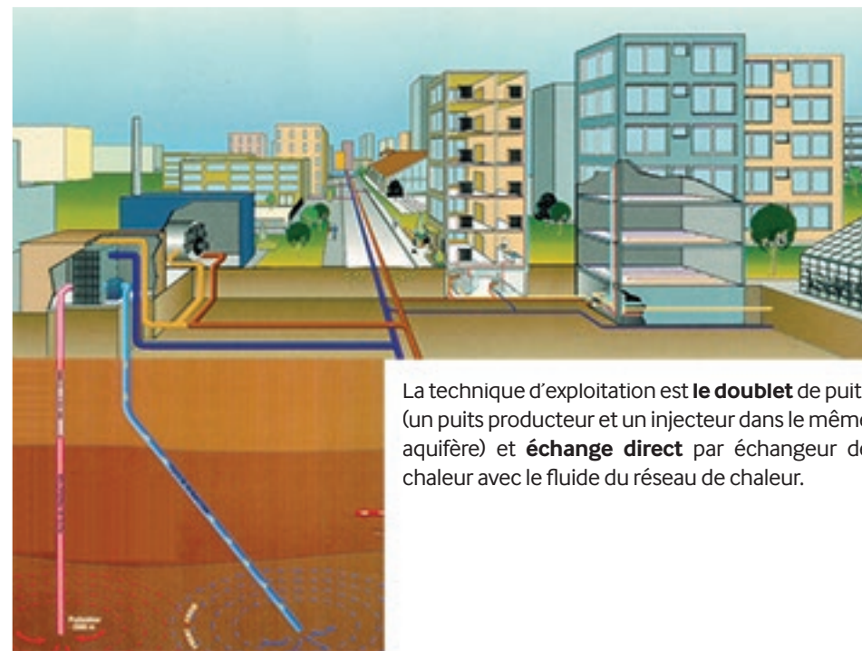
Géothermie profonde - Principe du doublet de puits
