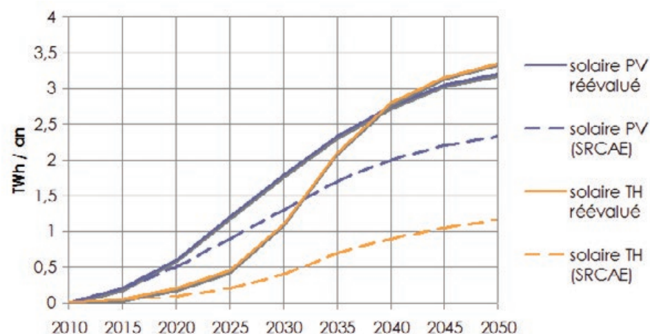
Évolution des productions solaires en Région Centre 2010-2050
