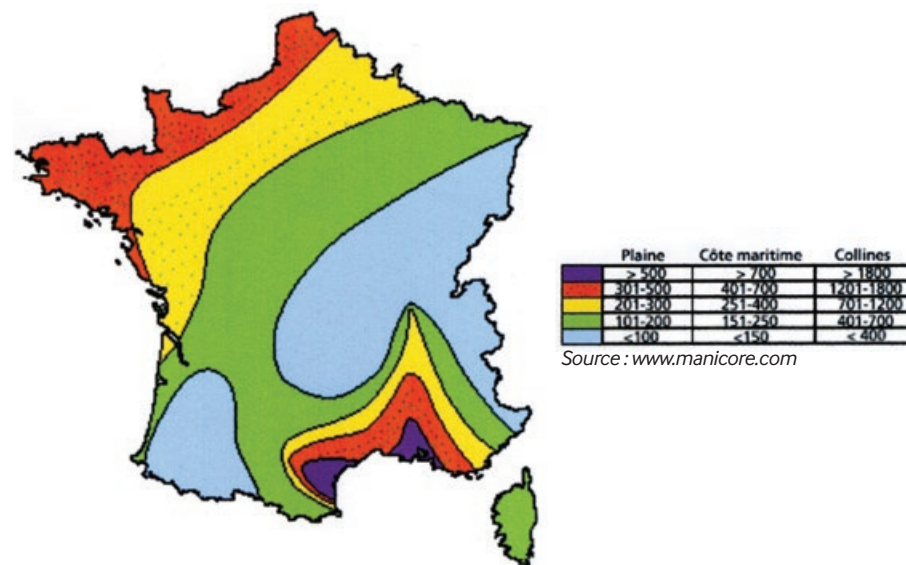
Figure 2 : Régimes des vents en France
