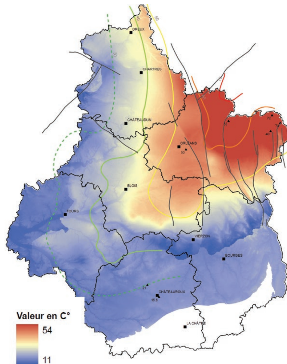
Carte de température des eaux du Dogger en région Centre (Source SRCAE)
