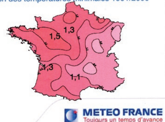
Evolution des températures minimales 1901/2000
