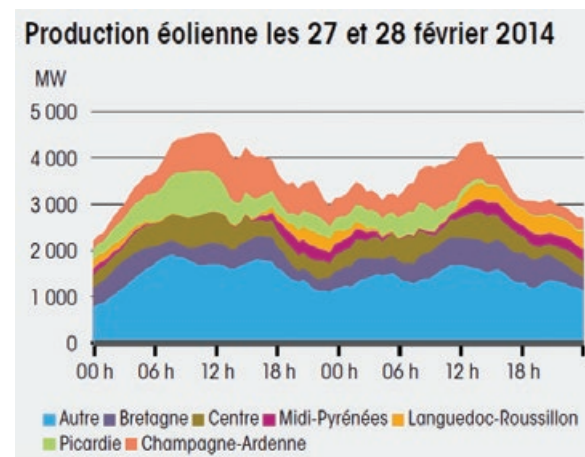
Figure 2 : L'observation des productions régionales montre l'absence de corrélation à l'échelle nationale. Ici, les régions Picardie et Languedoc Roussillon sont décorréliées.
