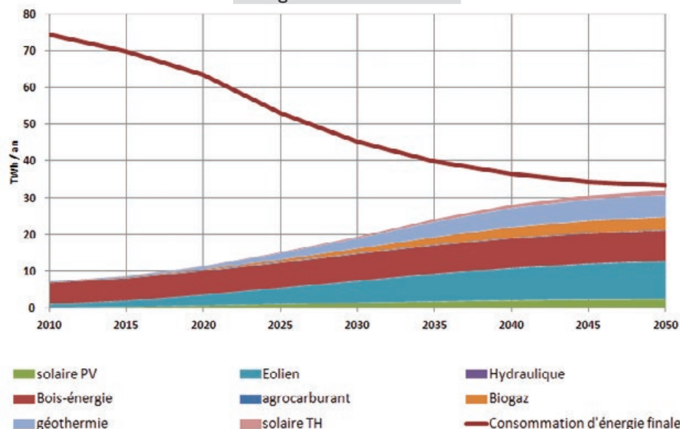
Évolution de la production et consommations énergétiques en Région Centre 2010-2050
