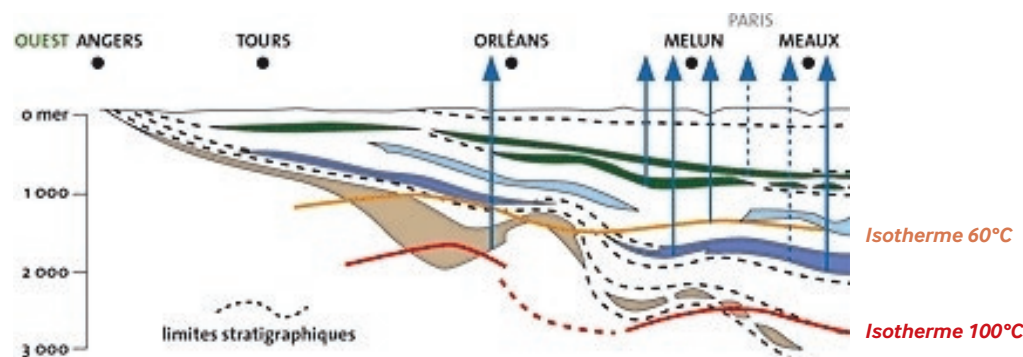
Coupe géologique du bassin parisien passant par Pithiviers, Orléans, sud de Blois, Tours et Angers (Source SRCAE région Centre)
