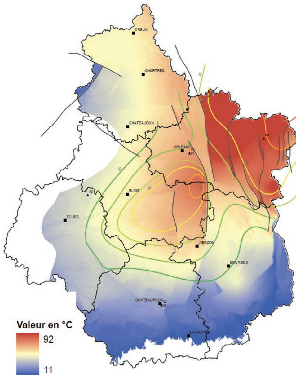
Carte de température des eaux du Trias en région Centre (Source SRCAE)
