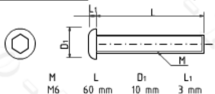
VIS A TETE PLATE (ici avec une encoche à 6 pans)
