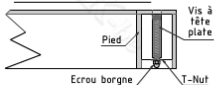
COUPE D'UN COIN DU MODULE
