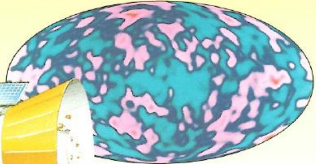
La carte micro-ondes établie par le satellite COBE.
