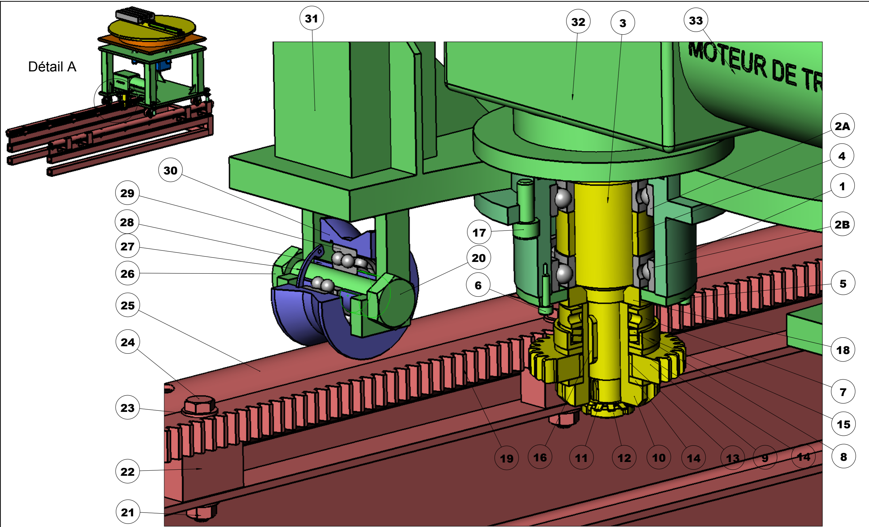
Vue de détail A
