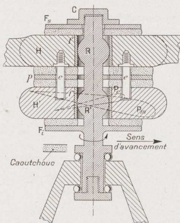
Rotor à 4 pales du clinogyre. Coupe possible du moyeu (interprétation de l'auteur).
