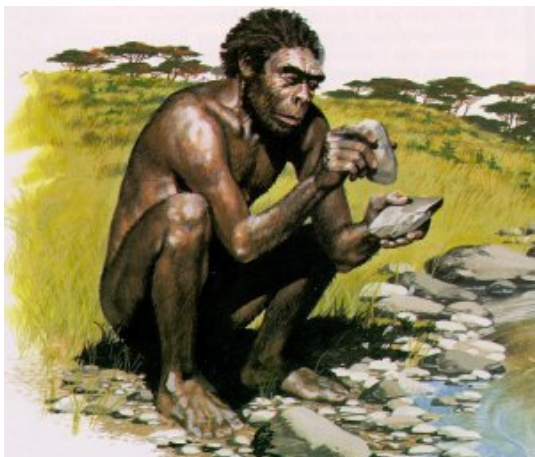
Homo habilis
