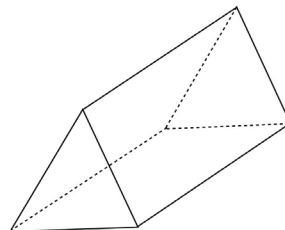
prisme
