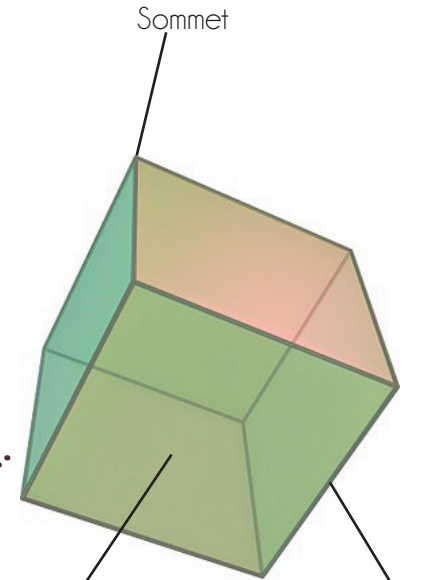
Arête
