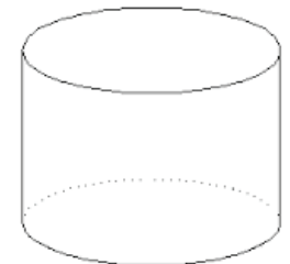
cylindre
