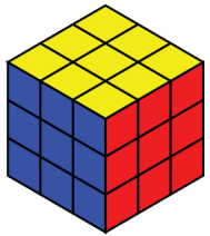
Polyèdre
