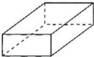
pavé droit
