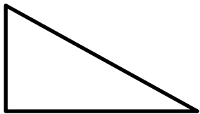
Les hauteurs d'un triangle
