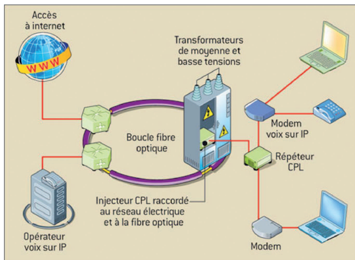
Exemple de réalisation : réseau local CPL
