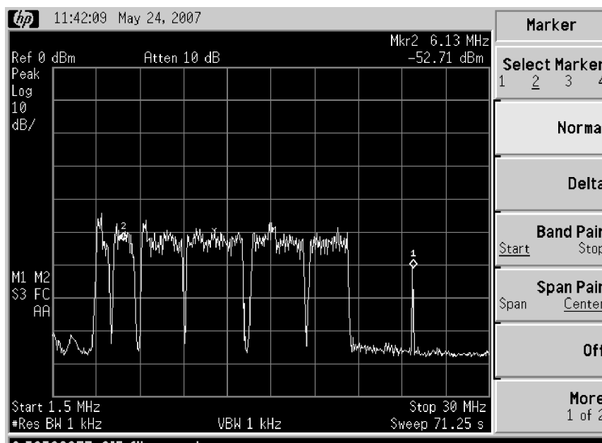
Spectre fréquentiel émis par un modem CPL
