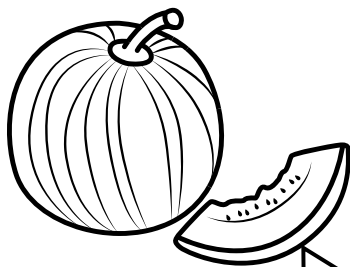
a melon
