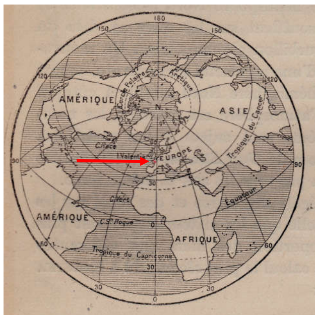
Figure 37 – Représentation de l’Hémisphère des Terres Émergées ou Hémisphère Continental selon Ritter corrigé de Penck ( Die Pole der Landoberfläche , pp. 121-126) et figuré par E. De Martonne, avec, fléché en rouge, son centre à proximité de Nantes.
