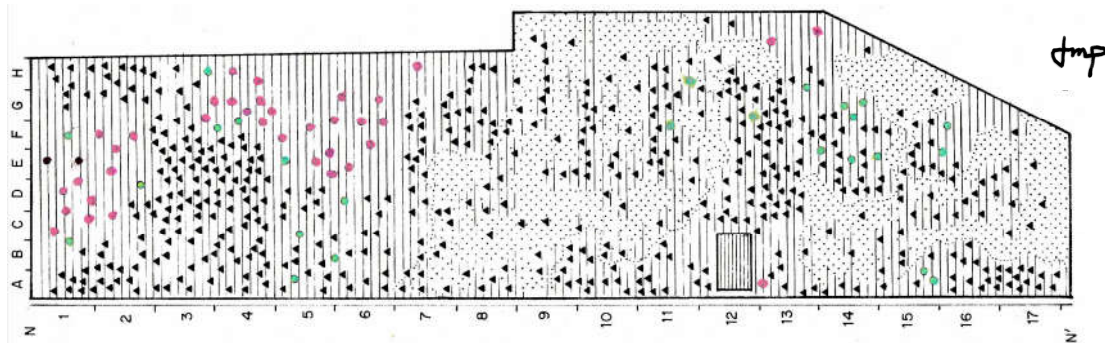
Parcelle de pins sylvestres (Gâvre – v. plan général p. SP V) triangles noirs = pins – points verts = chênes vivants – points roses = chênes morts pointillé = Myrica gale – hachures = Molinia caerulea surface plantée approchée = 2500 m 2
