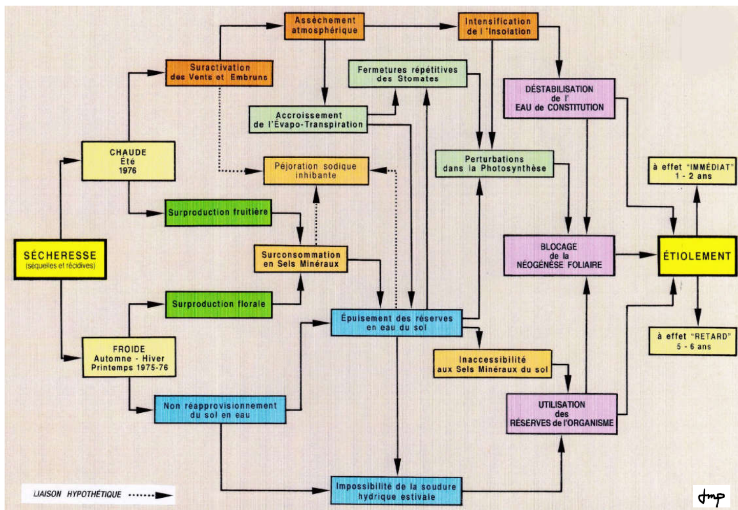
Figure 38 – Les mécanismes létaux (étiollement) de la végétation arborée en période caniculaire aride (observés, mesurés et analysés en forêt littorale dunaire vendéenne)
