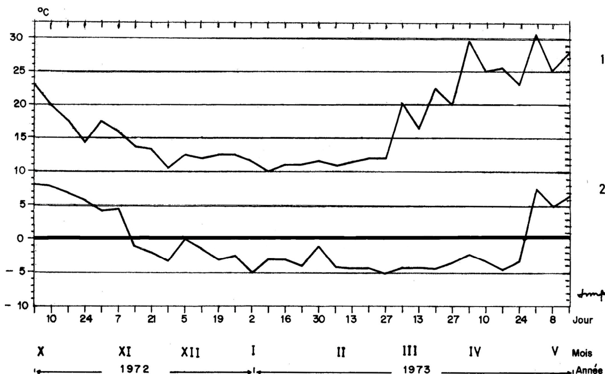
Thermogramme des maxima (1) et des minima (2) absolus, hebdomadaires sous pineraie sylvestre figurée en aplat lilas dans le relevé d'ensemble d'un milieu humide forestier (p. SP V) et dans le plan détaillé de la page 223.b
