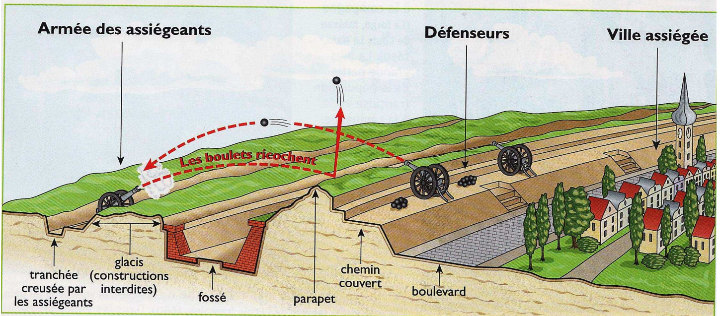
Doc. 2 Coupe d'une fortification de Vauban.
