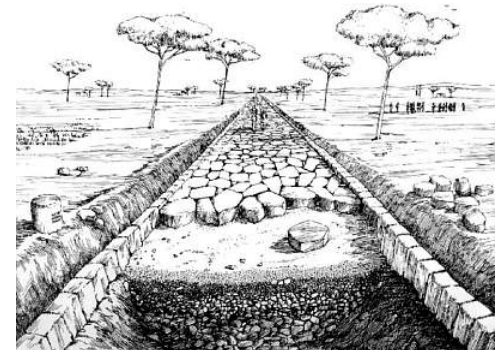
Croquis en coupe d'une voie romaine.
