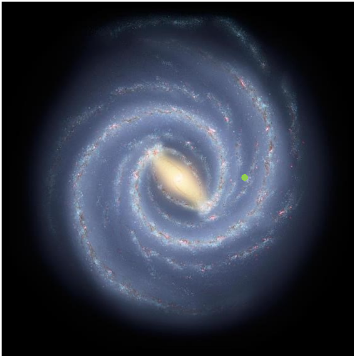
Voie lactée
