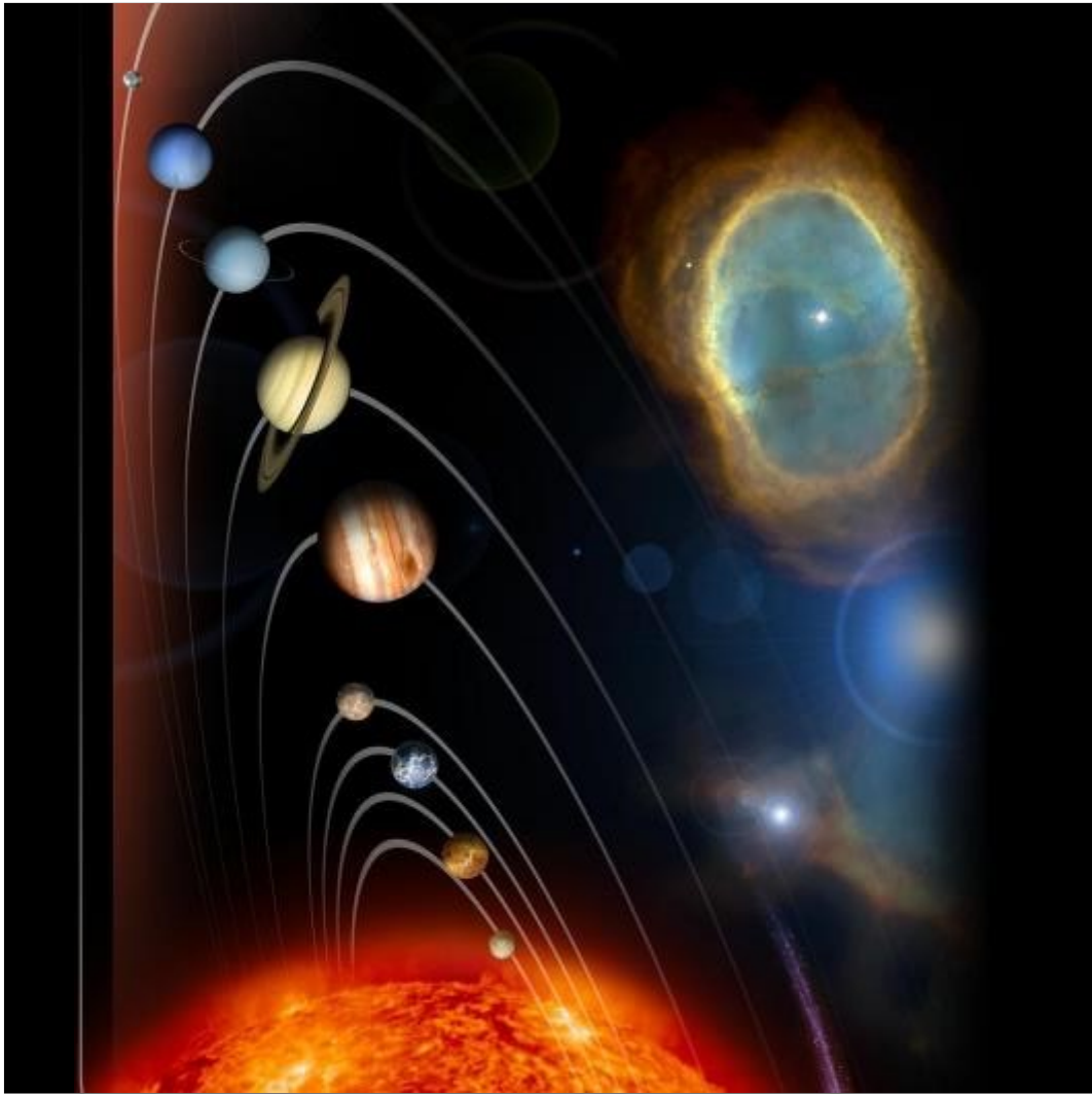
Système solaire
