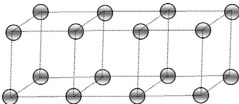
Arrangement périodique d'atomes dans un cristal
