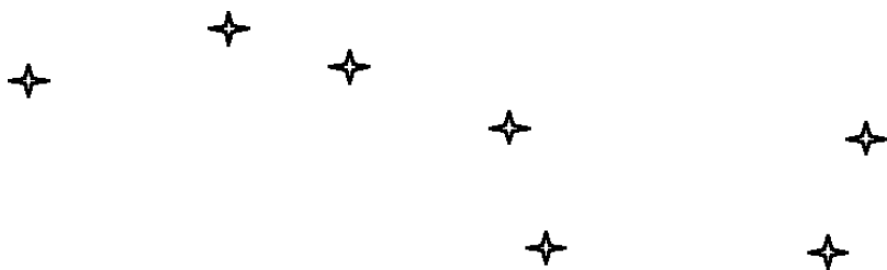
La Grande Ourse
