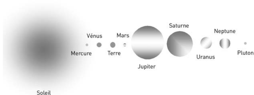
Les 9 planètes du système solaire et leur taille relative
