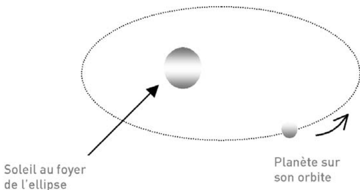
La trajectoire des planètes autour du Soleil
