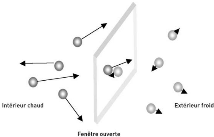
L'agitation des molécules selon la température
