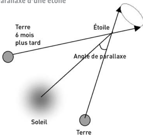
Parallaxe d'une étoile
