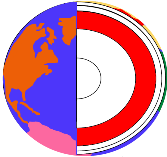
manteau inférieur
