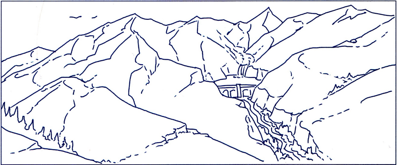
▲ une montagne jeune
