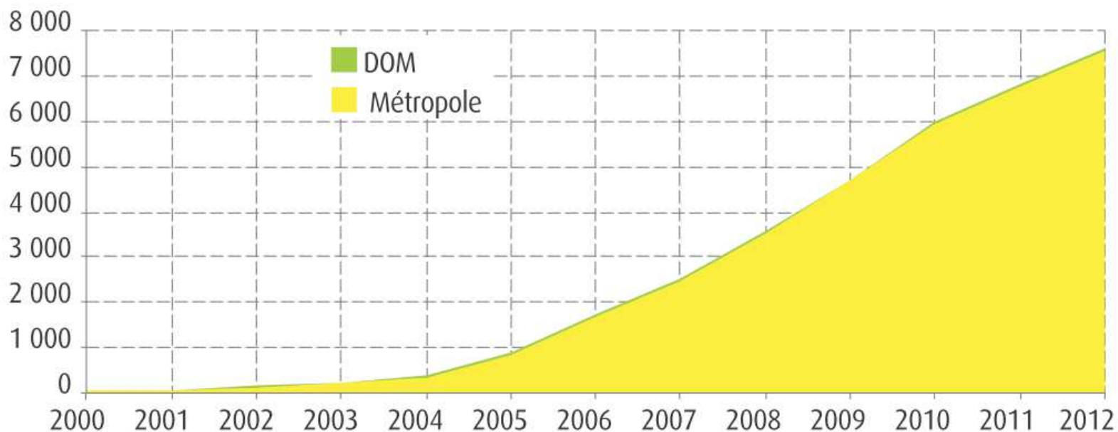
Solaire photovoltaïque: puissance installée en fin d'année, en MW
