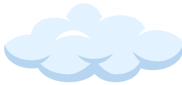
le nuage
