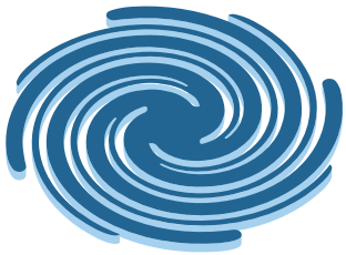
le cyclone
