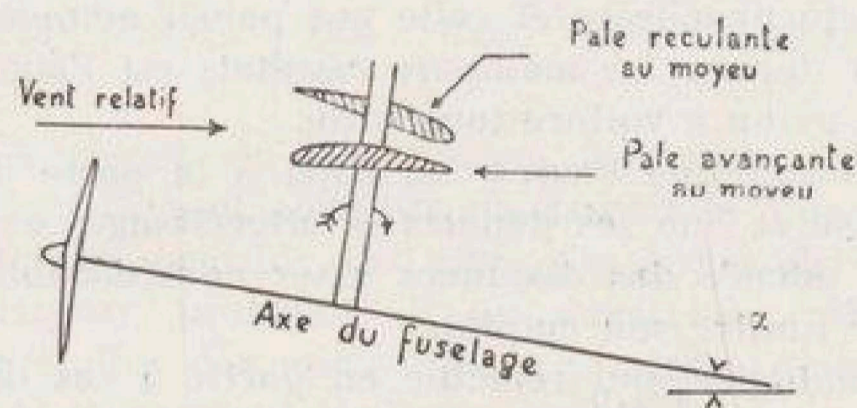
Schéma de la voilure du clinogyre
