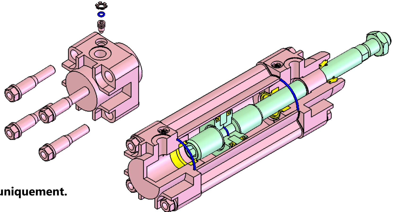
Système de réglage de l'amortissement
