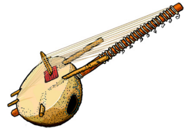
Une kora
