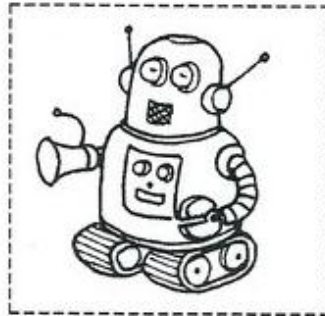
un robot
