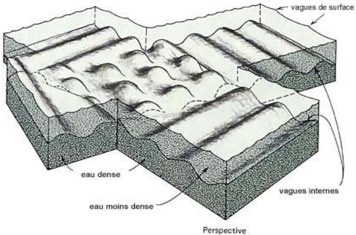
Illustration 16: Vagues internes sur l'interface située entre deux couches d'eau de densités différentes. L'une est dense (celle du bas), alors que l'autre est moins dense (celle du haut). ( Oceanography [L'océanographie], Gross, p. 204.)
