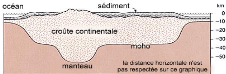
Illustration 7: Les montagnes ont de profondes racines sous la surface de la terre. ( Earth [Terre], Press et Siever, p. 413.)
