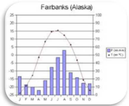
Diagramme ombrothermique
