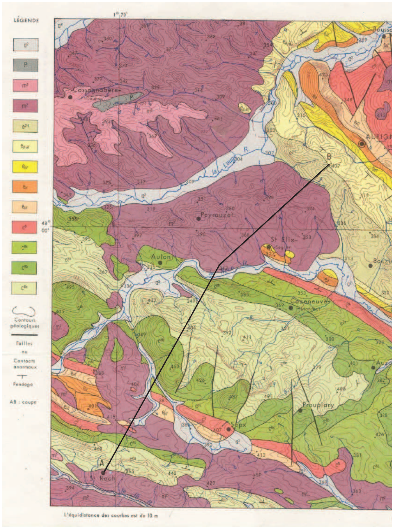
Document 1 : extrait de la carte géologique de St Gaudens au 1:50000
