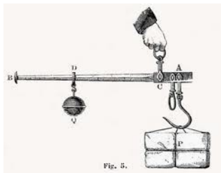
balance romaine
