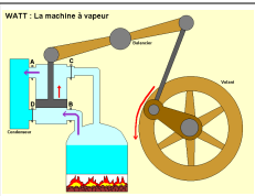
Machine à vapeur
