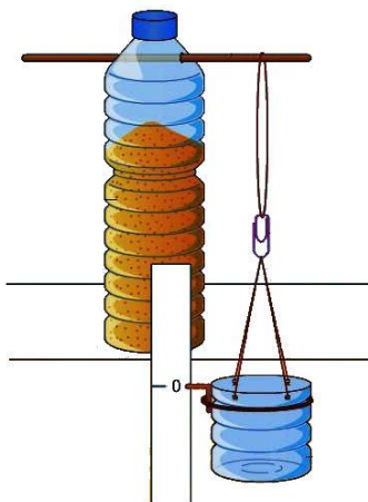
Balance à élastique
