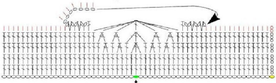
Dessus
