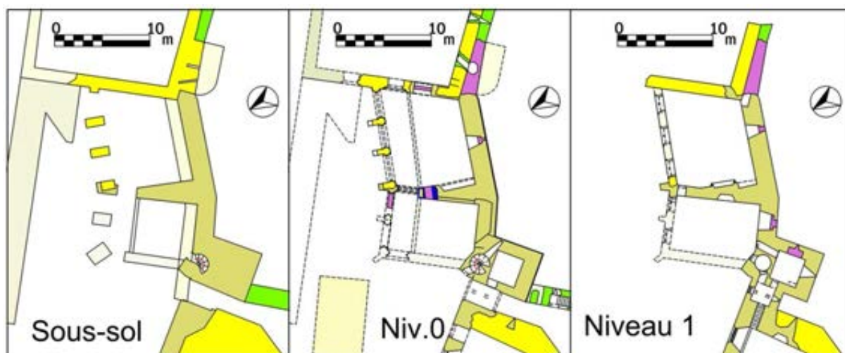
Figure 37: Plans de la Chambre aux chevaliers à ses différents niveaux
