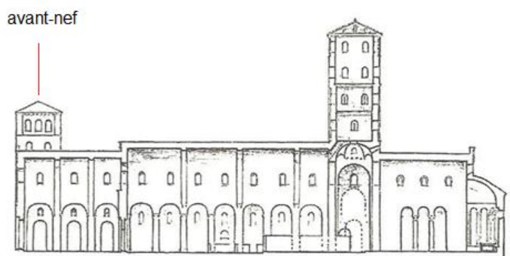
Fig.1 - Coupe longitudinale de Cluny II 55
